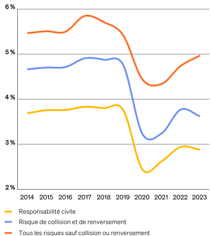
Fréquence des réclamations pour les voitures de tourisme (pourcentage)
